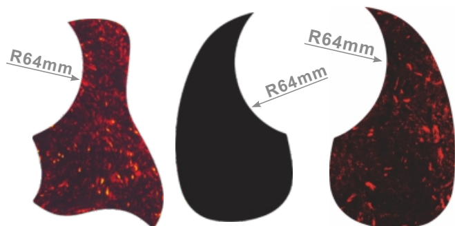
A025F 彩色护板
